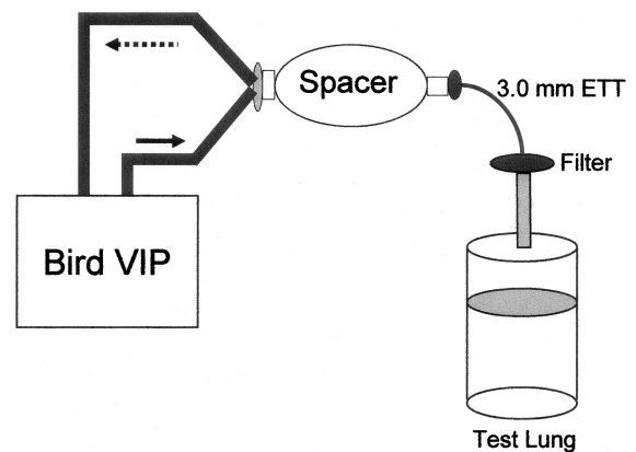
Fig. 1. Neonatal ventilator-lung model. ETT = endotracheal tube.
